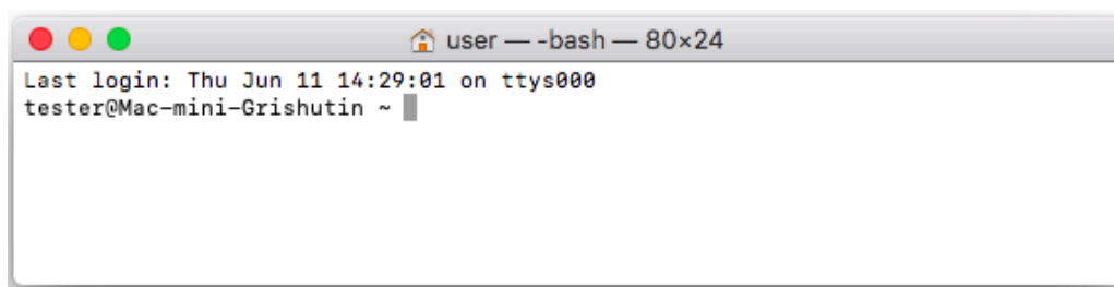
Рис. 4.6. Вікно Терміналу
